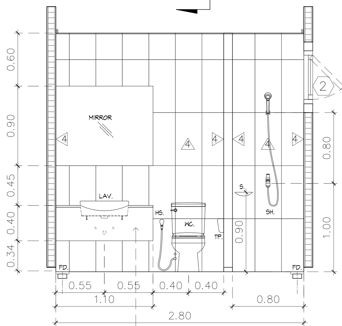
รูปตัด 1 SCALE 1:25
