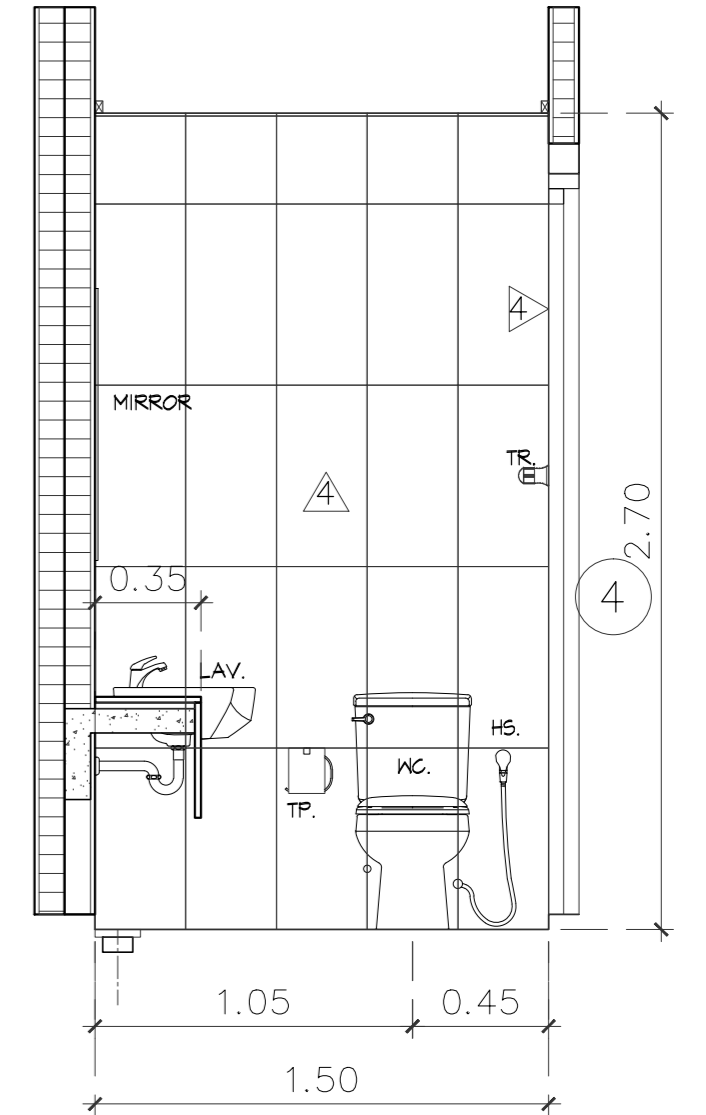
รูปตัด 2 SCALE 1:25
