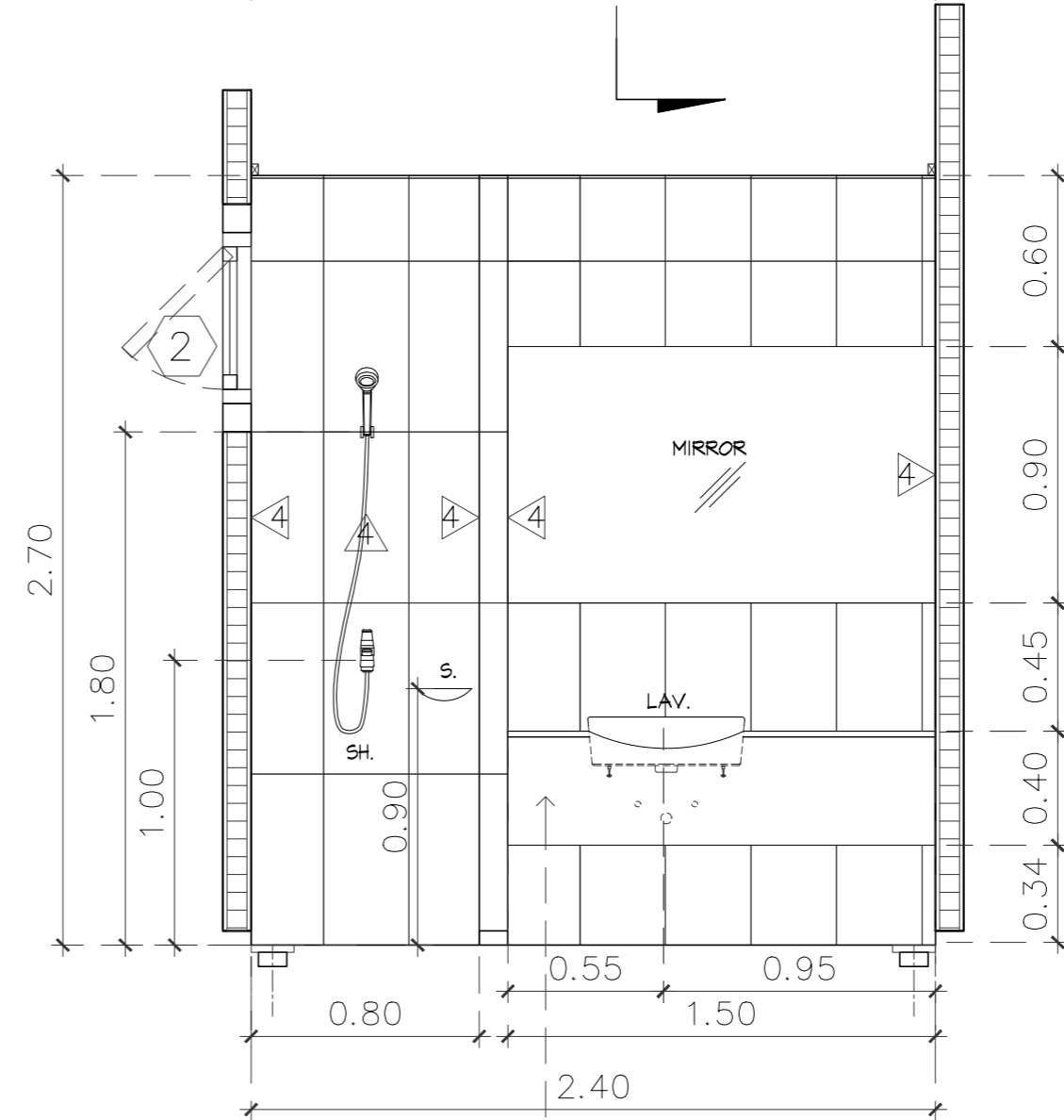
รูปตัด 1 SCALE 1:25
