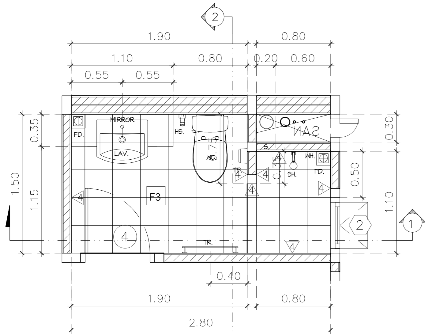
แปลนขยายห้องน้ำ 1 SCALE 1:25
