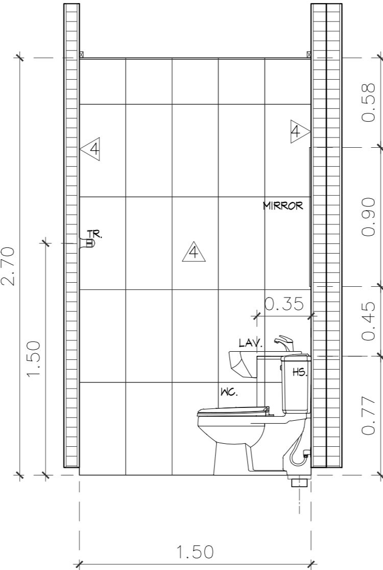
รูปตัด 2 SCALE 1:25
