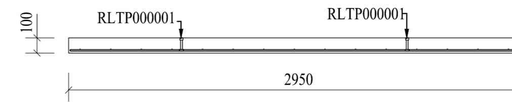
B-B (1:25)
