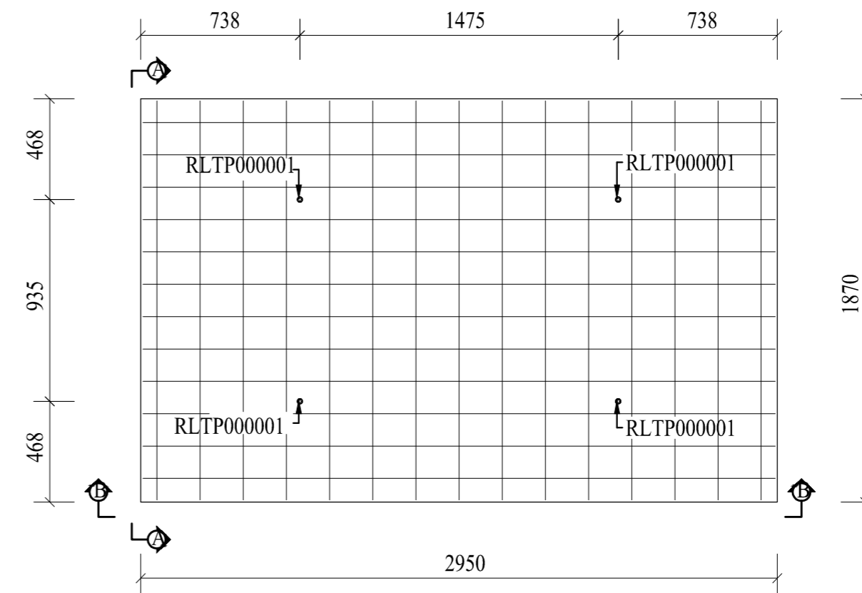
Plan (1:25)
