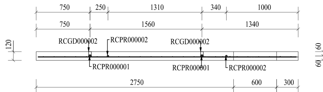
B - B (1:25)
