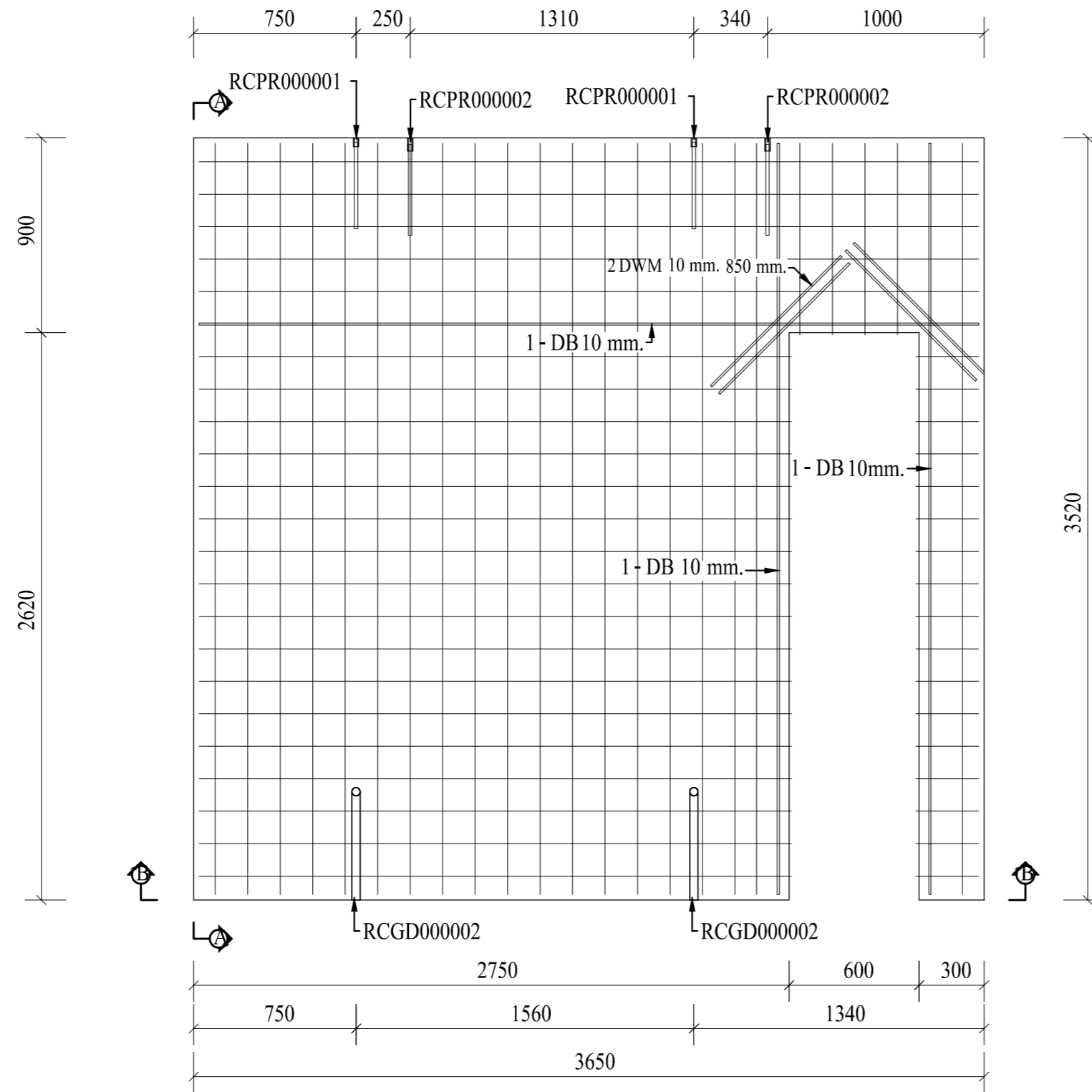
Plan (1:25)
