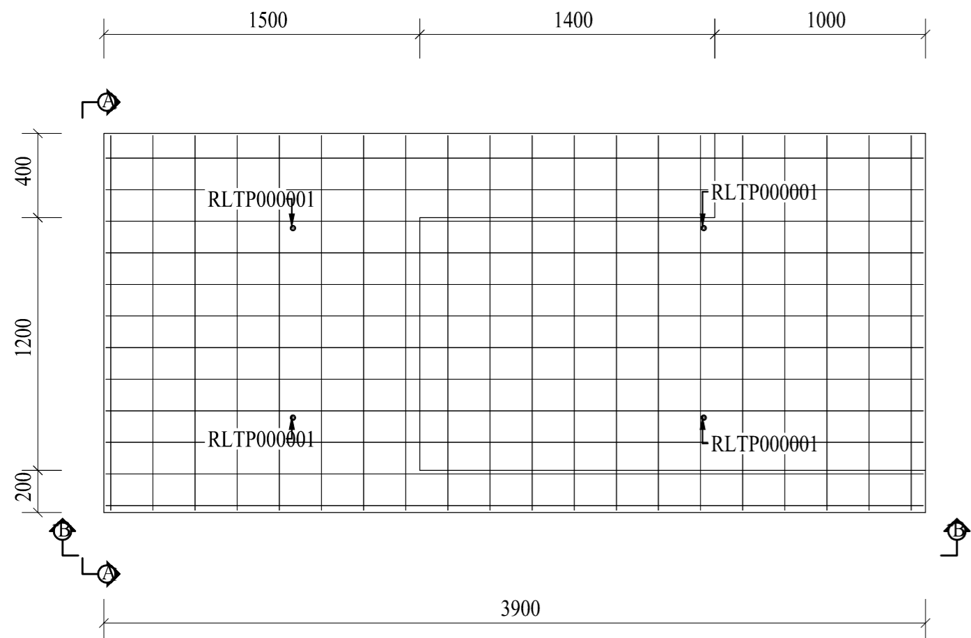
Plan (1:25)
