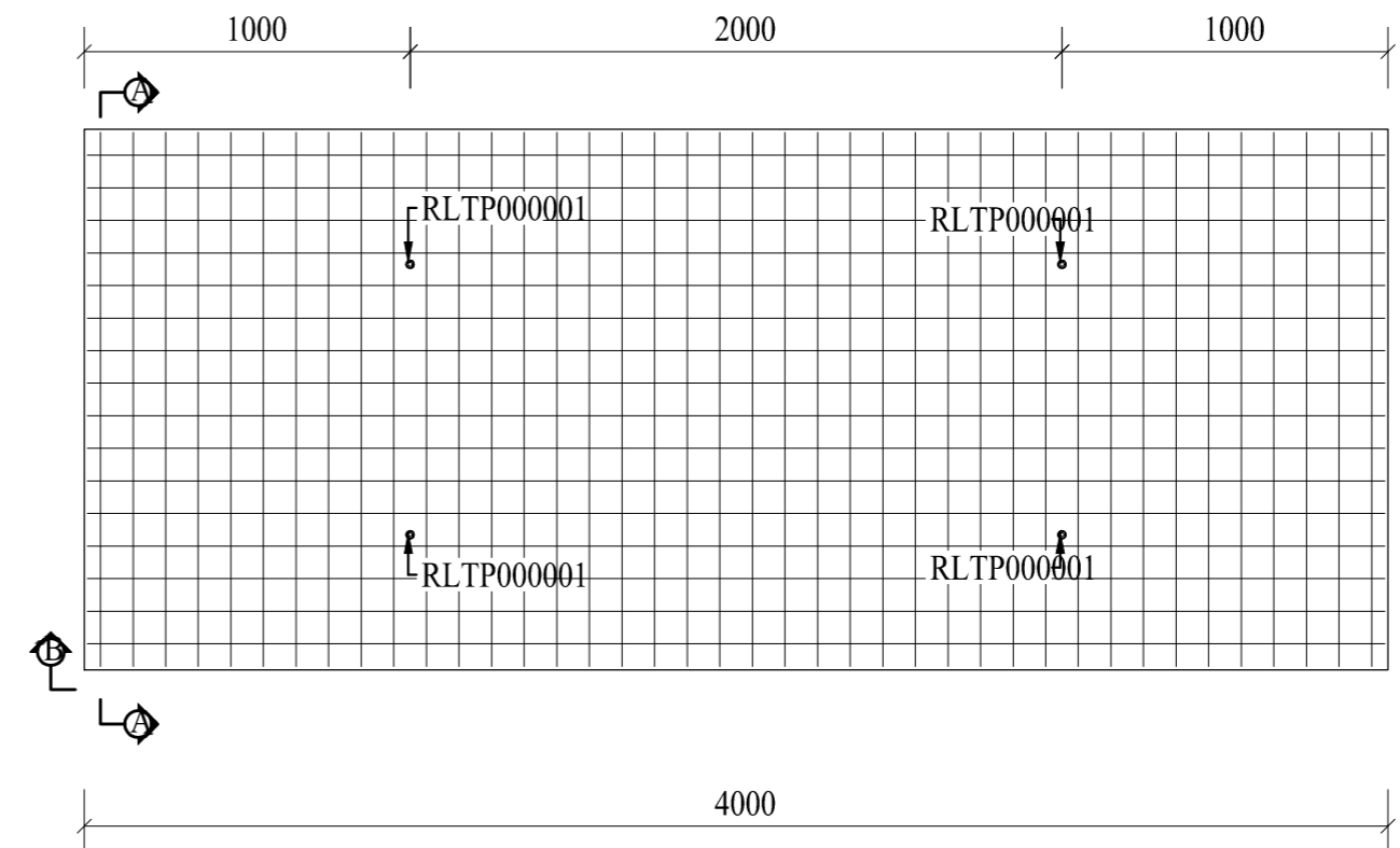
Plan (1:25)
