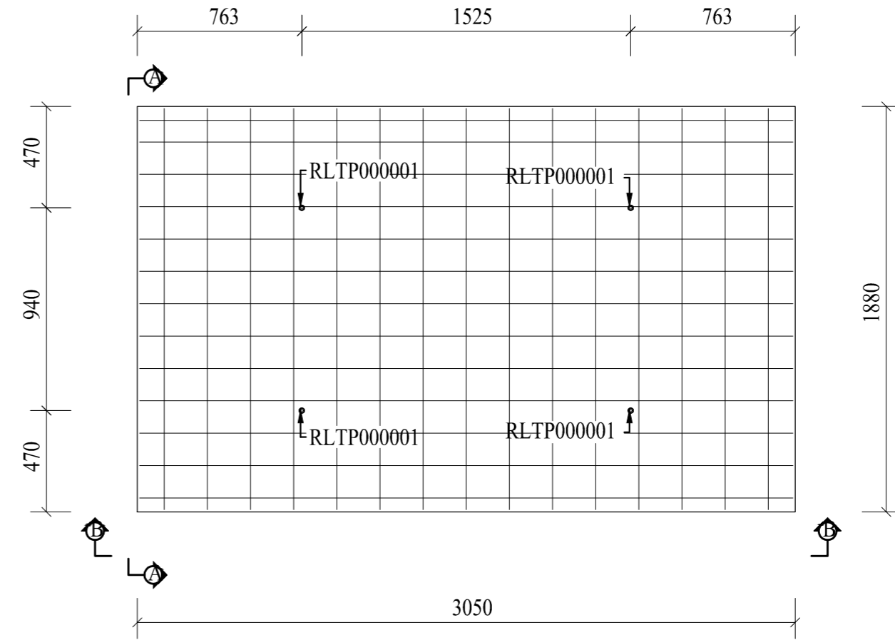
Plan (1:25)
