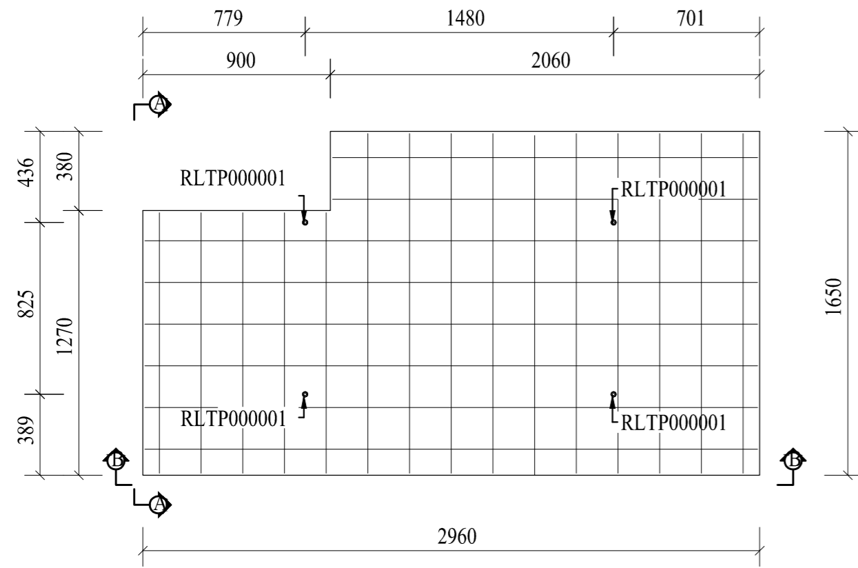
Plan (1:25)
