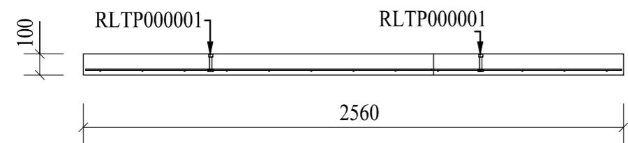
B-B (1:25)
