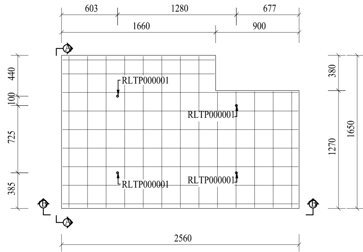
Plan (1:25)
