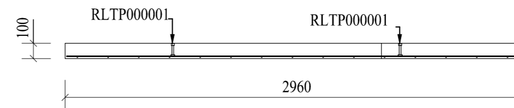
B-B (1:25)
