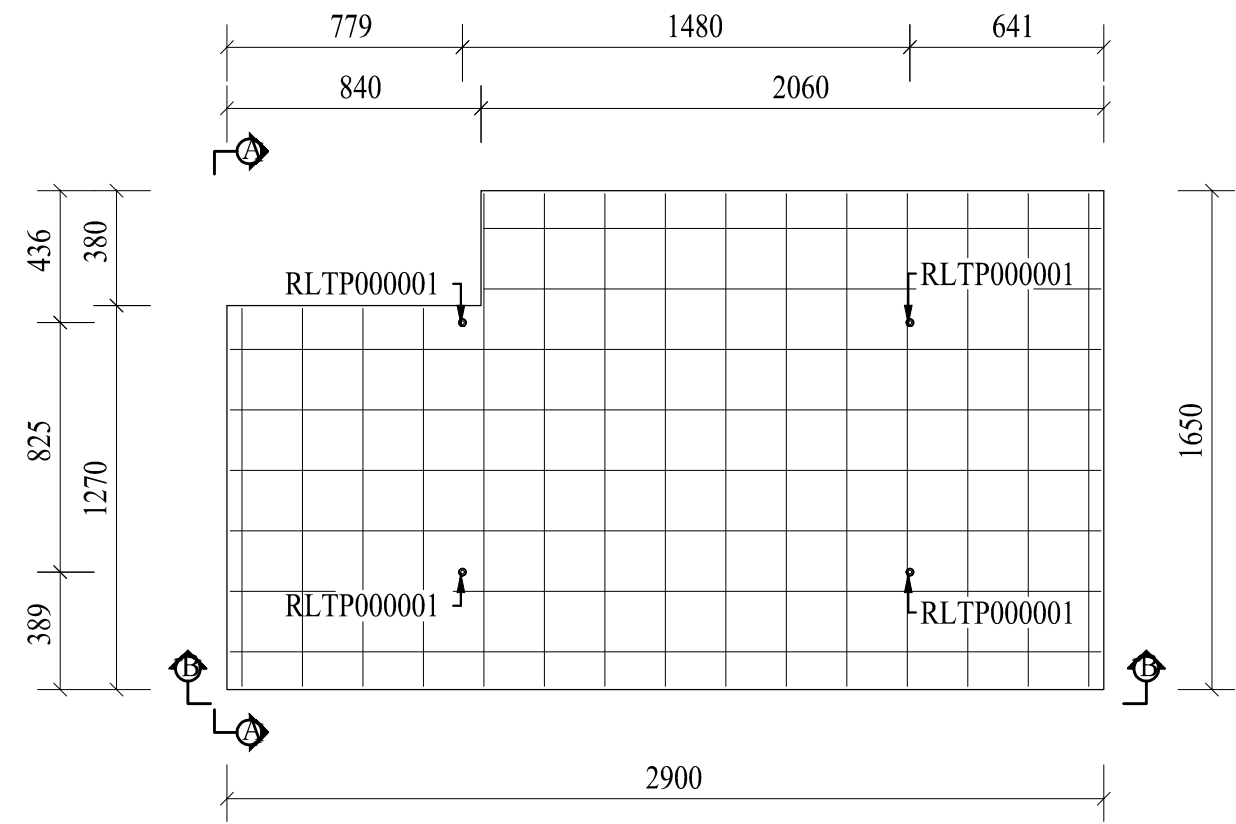
Plan (1:25)
