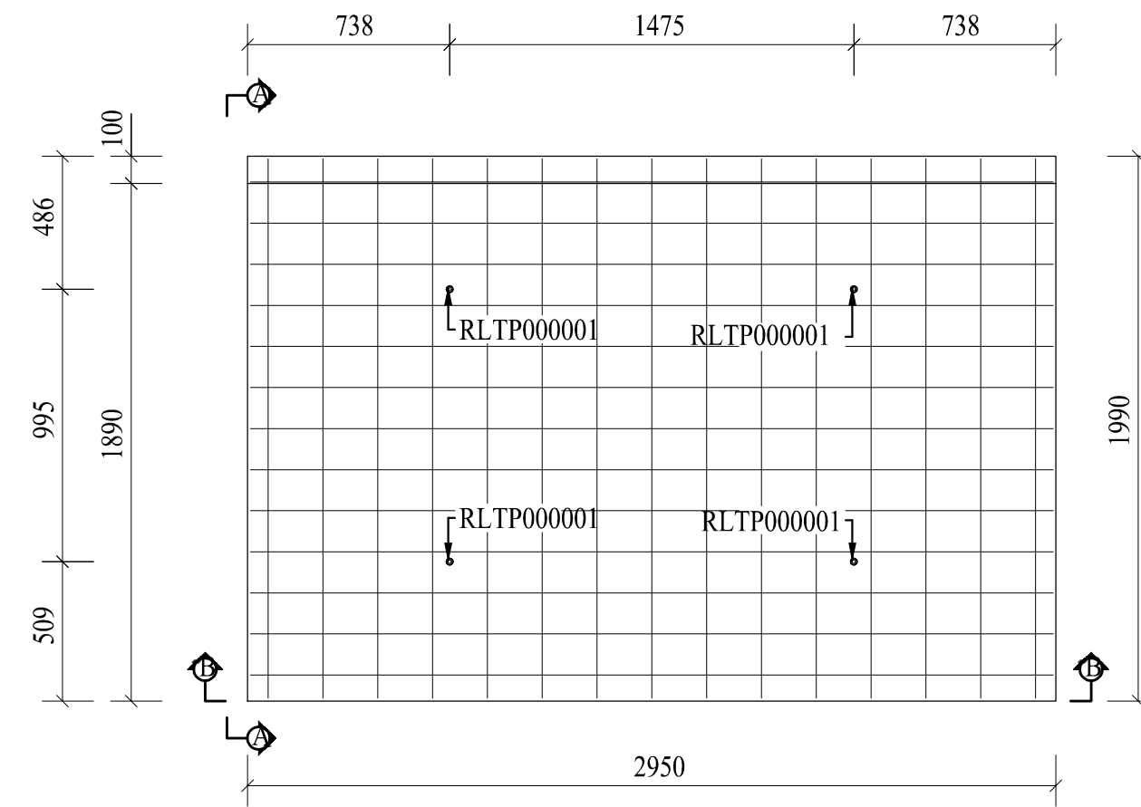
Plan (1:25)
