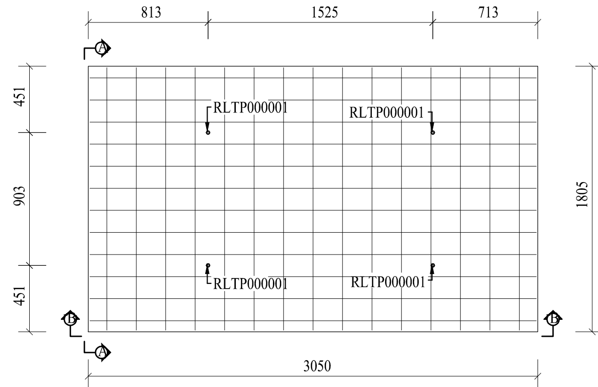
Plan (1:25)
