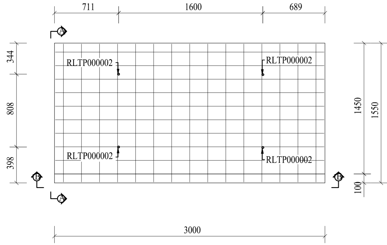
Plan (1:25)
