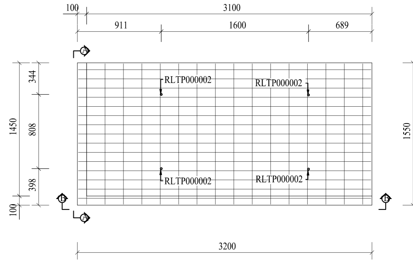
Plan (1:25)
