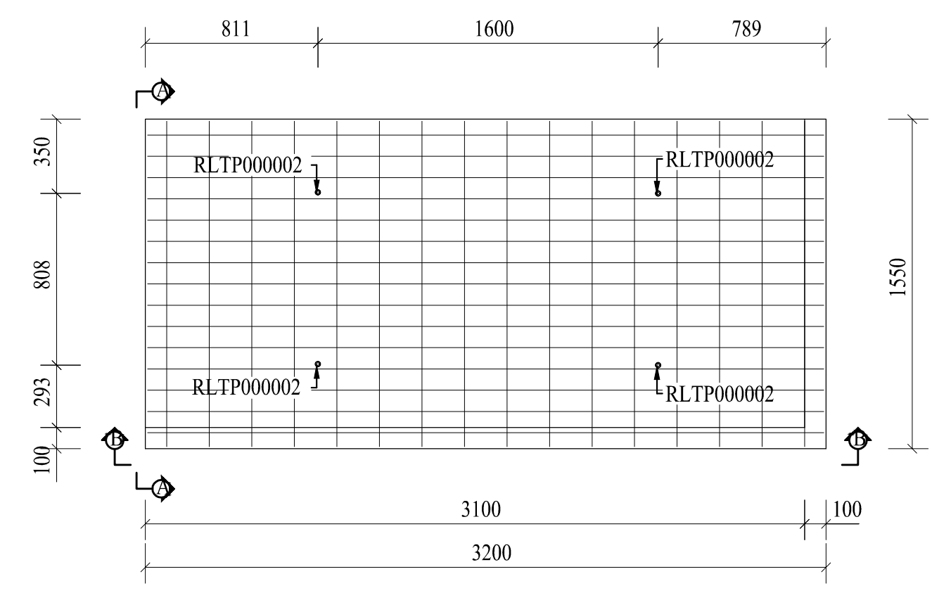
Plan (1:25)
