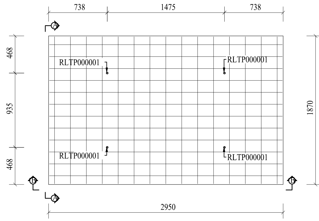
Plan (1:25)
