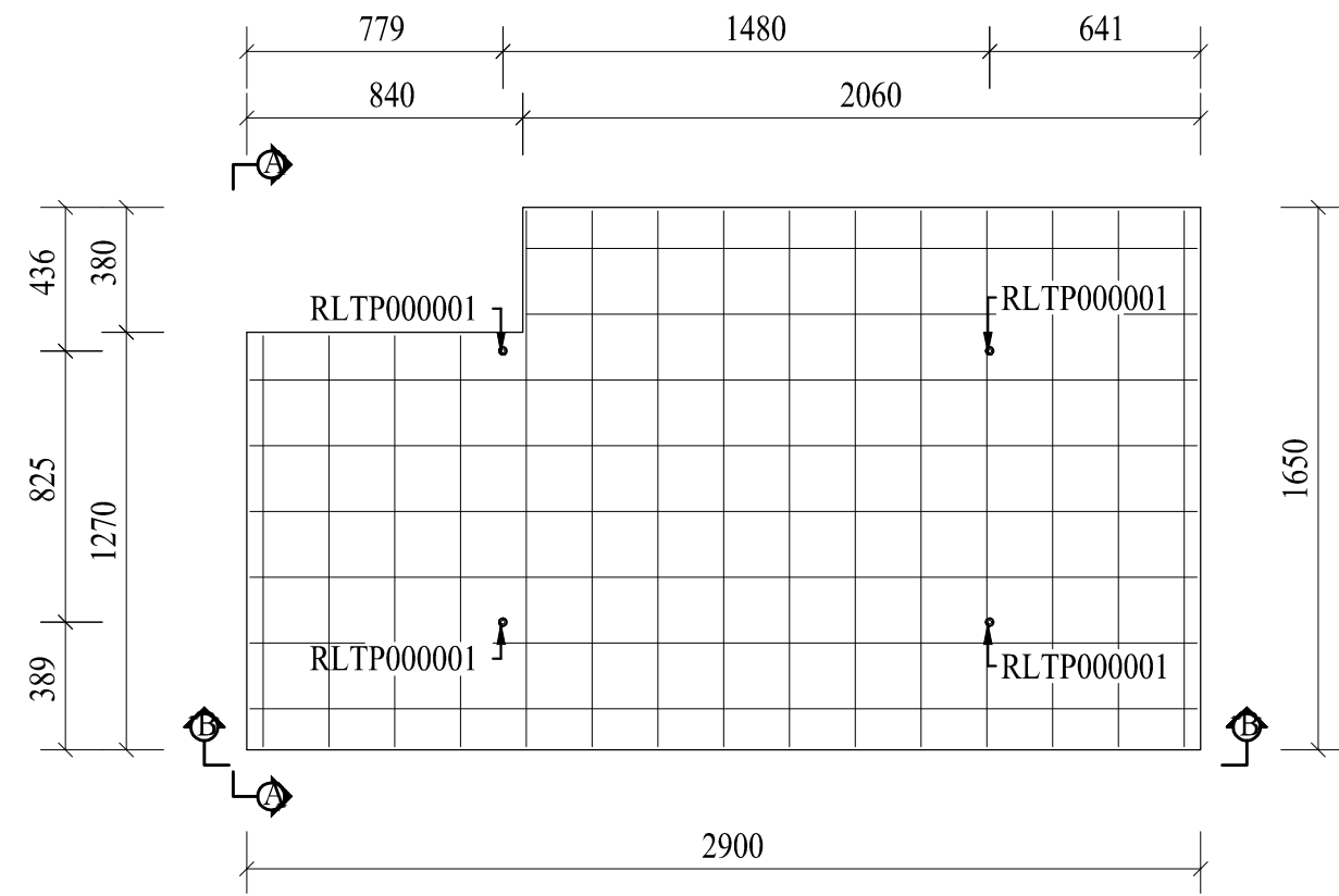
Plan (1:25)
