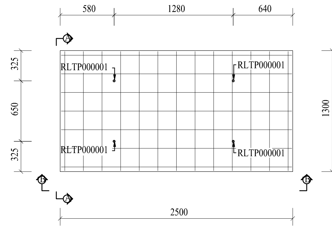
Plan (1:25)
