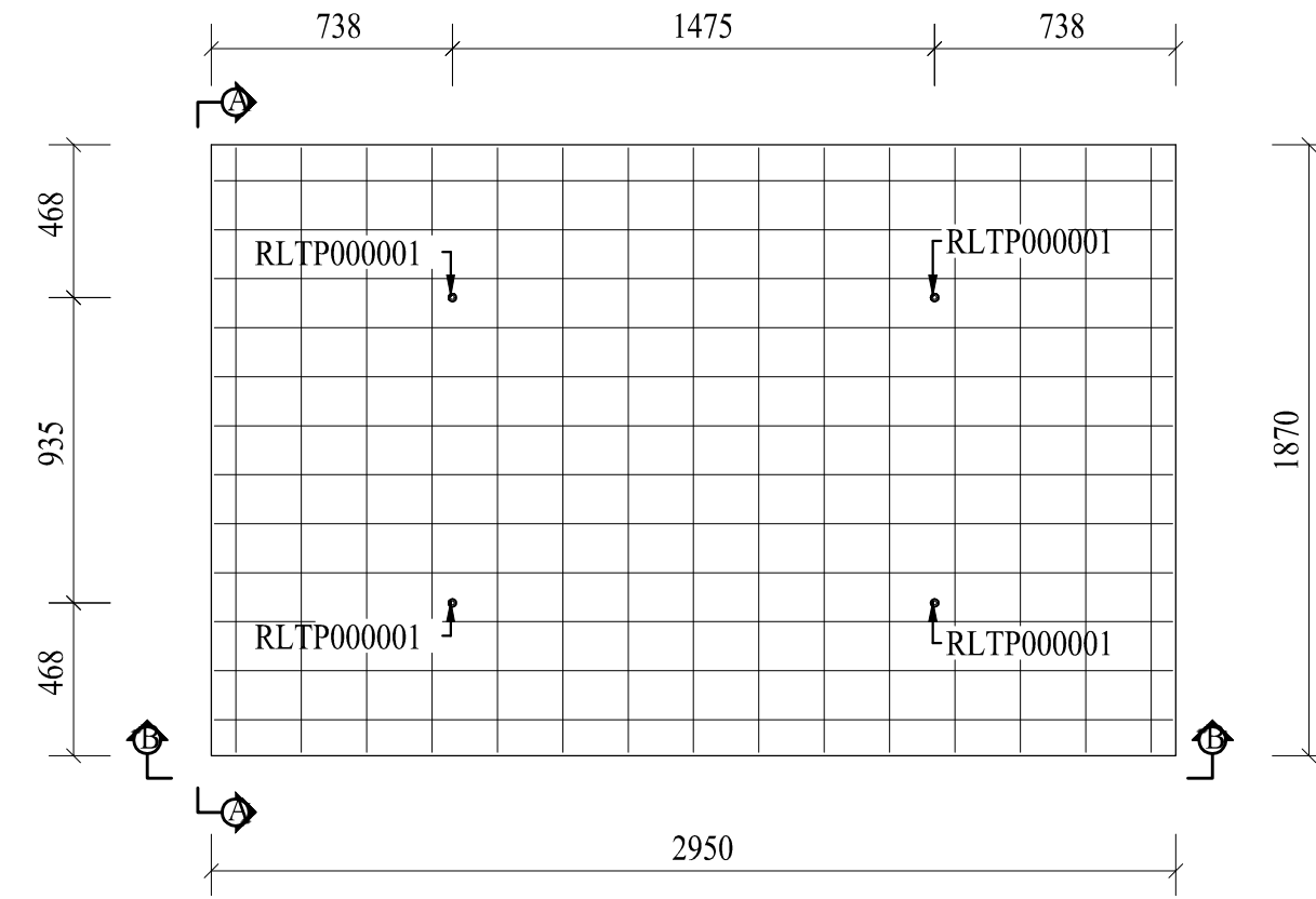
Plan (1:25)
