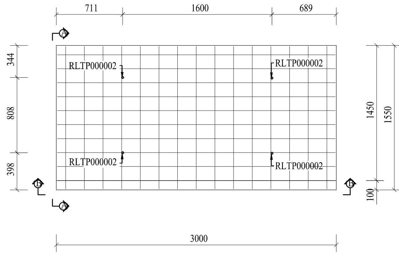
Plan (1:25)
