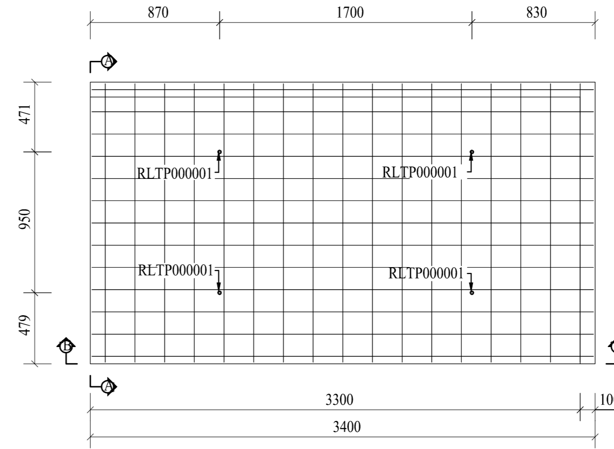
Plan (1:25)
