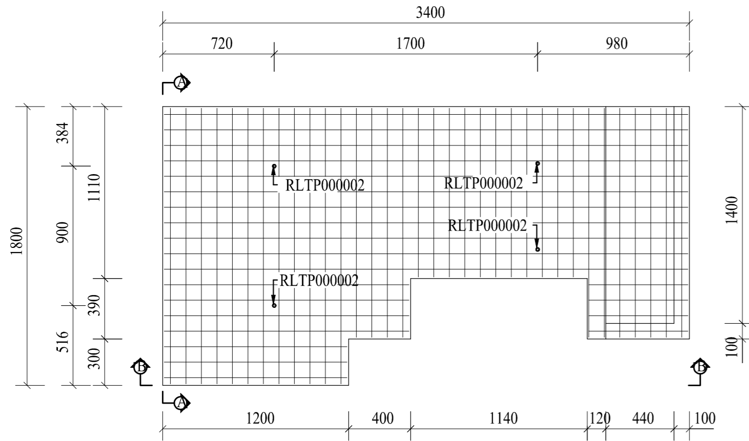
Plan (1:25)
