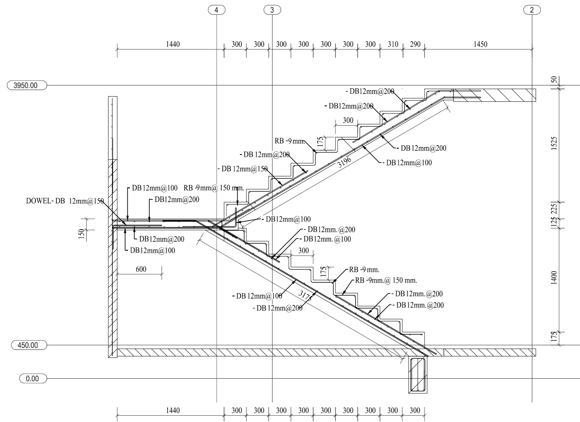
ขยายบันไดหนีไฟ (1:25)
