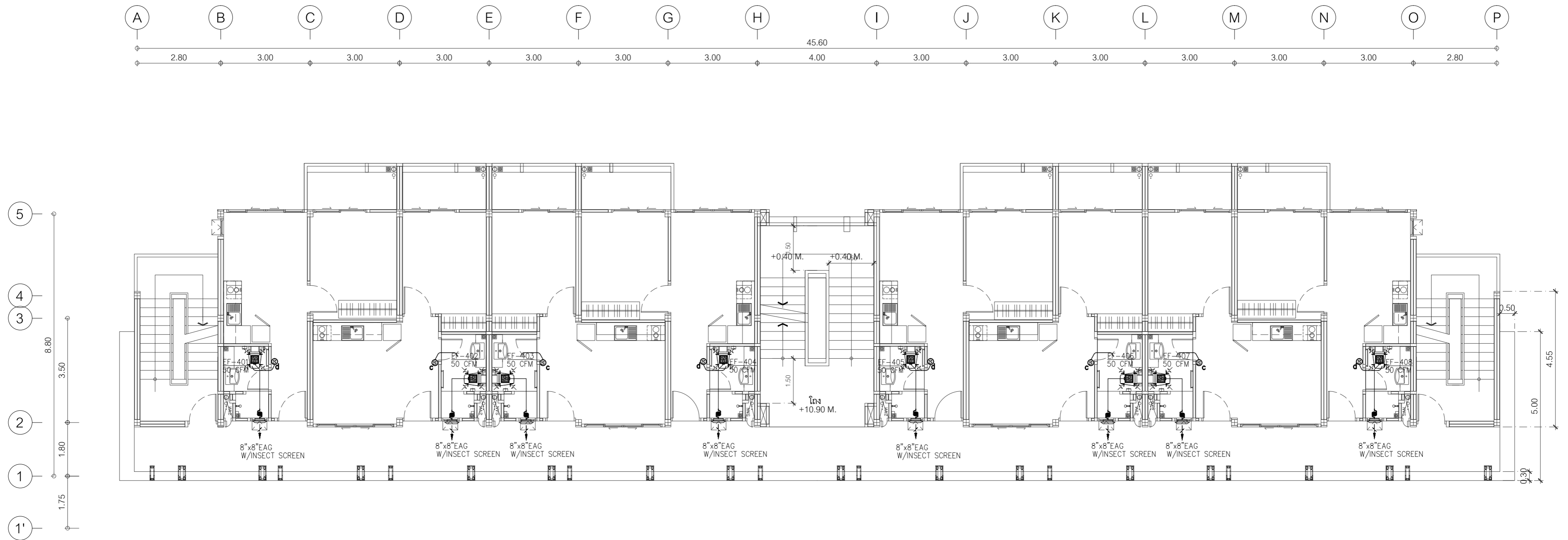
แปลนระบบปรับอากาศและระบายอากาศชั้น 4 SCALE 1:100
